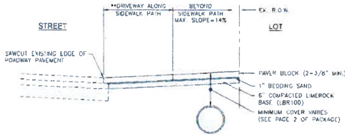
SECTION C N.T.S.
