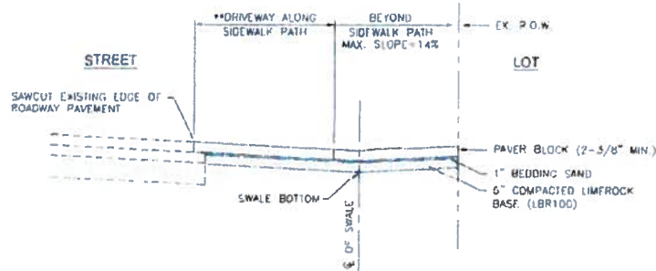
SECTION D N.T.S.
